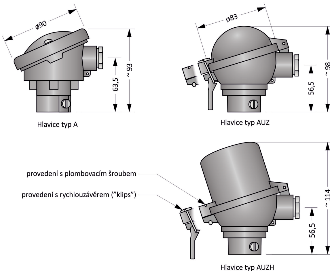
Obrázek 2L.2: Typy hlavic
