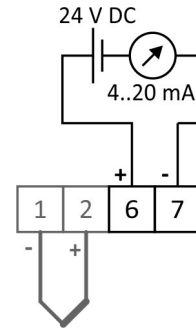
Obrázek 2L.3: zapojení převodníků
