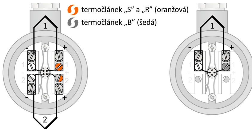
Obrázek 2L.4: zapojení dvojitého termočláňku
